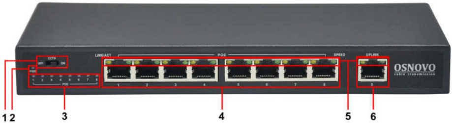
Рис. 2 Коммутатор SW-20900/В, разъемы и индикаторы на передней панели
